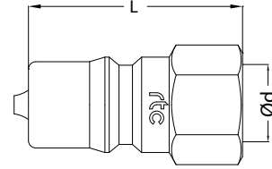
Female Thread Plug / Nippel mit Innengewinde
