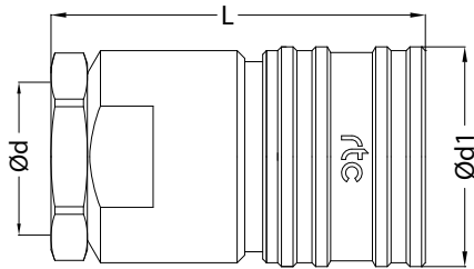
Female Thread Socket / Kupplung mit Innengewinde
