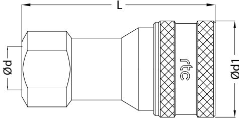
Female Thread Socket / Kupplung mit Innengewinde
