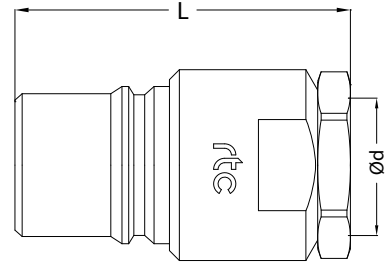
Female Thread Plug / Nippel mit Innengewinde
